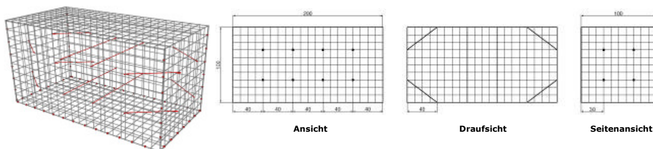
C-Klammer-Gabione , 200 x 100 x 100 cm, Masche 10 cm
