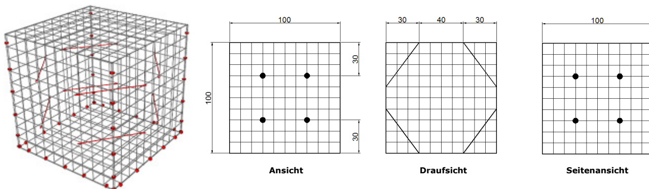
C-Klammer-Gabione , 100 x 100 x 100 cm, Masche 10 cm
