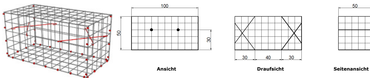
C-Klammer-Gabione , 100 x 50 x 50 cm, Masche 10 cm
